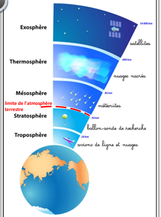
Atmosphère terrestre.
